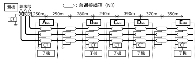
ケーブル種別: XLPE (CV)、電圧階級: 66kV、導体断面積: 500mm 2 、遮蔽層構造: ワイヤシールド、接地方式: ソリッドボンド接地方式
