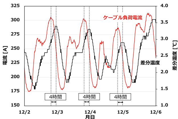
図6 ケーブル表面温度とMH内雰囲気温度との差分温度と負荷電流の変化
