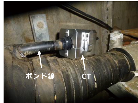
写真1 ボンド線または接地線へのCTの誘導結合例
