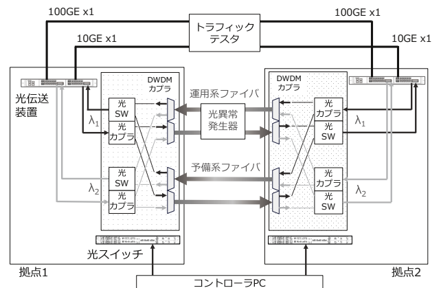
図9 冗長切替え性能評価構成
