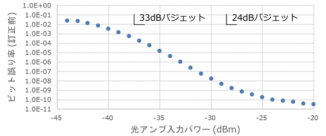
図7 100G受信誤り率 (誤り訂正前)
