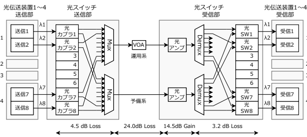
図6 伝送評価システム構成
