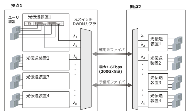
図5 システム構成例
