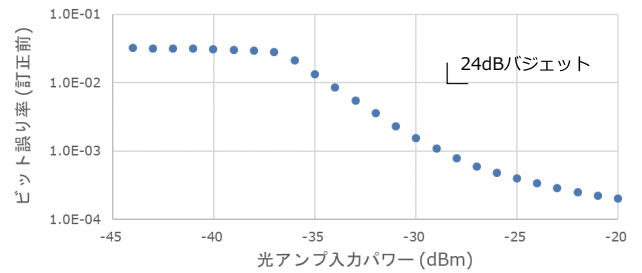
図8 200G受信誤り率 (誤り訂正前)
