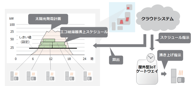
図5 エコ給湯機制御
