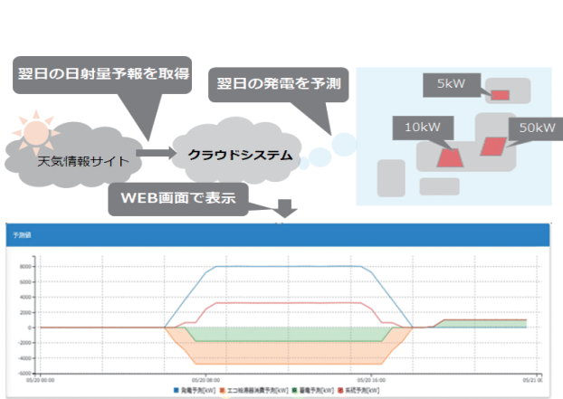
図3 太陽光発電電力予測
