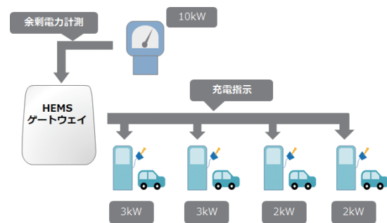
図6 EV充電器制御
