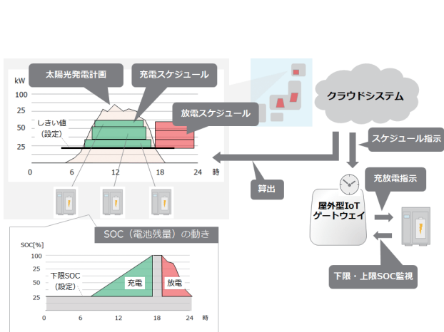
図4 蓄電池制御
