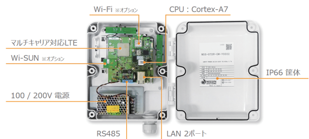
写真2 HEMSゲートウェイ
