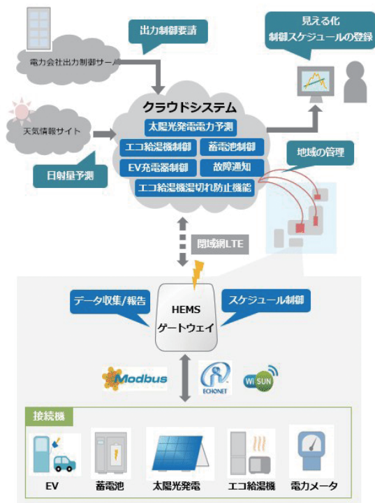
図2 SPSS-Hシステム構成
