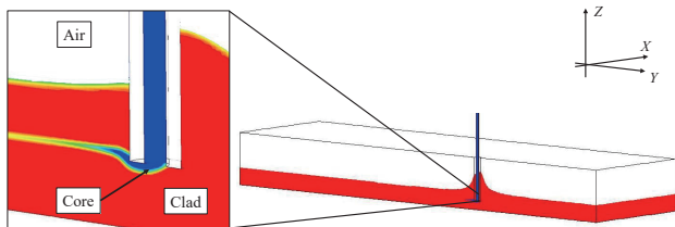
図5 モスキート法による導波路作製の流動解析モデル
