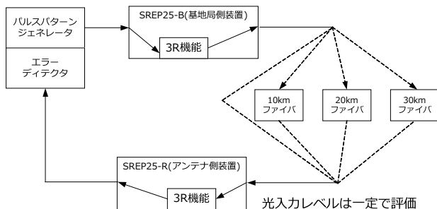
図7 選択した波長の距離に対する誤り率の測定系
