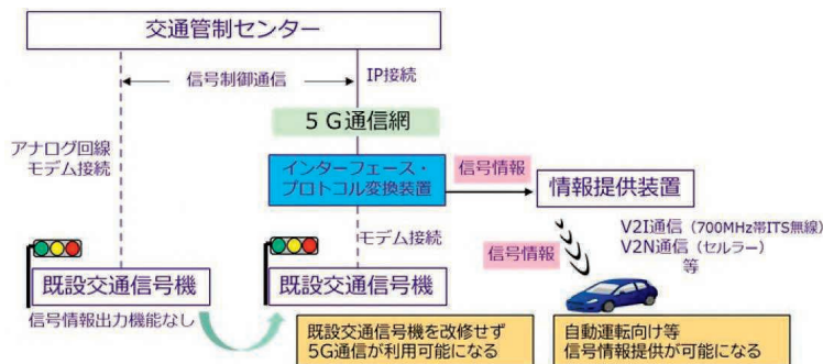
インターフェース・プロトコル変換装置の概要
