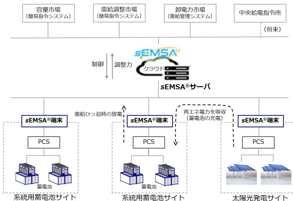
系統用蓄電池と sEMSA®を組み合わせたシステムイメージ
