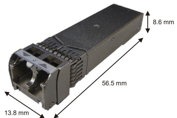
Photo 1. SFP28 module
